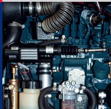
Motore Kubota 3600 rpm
